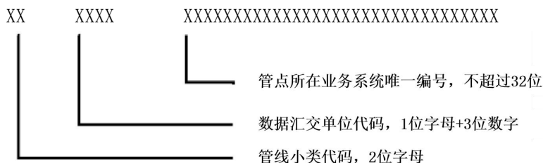
图 2 管点编码
