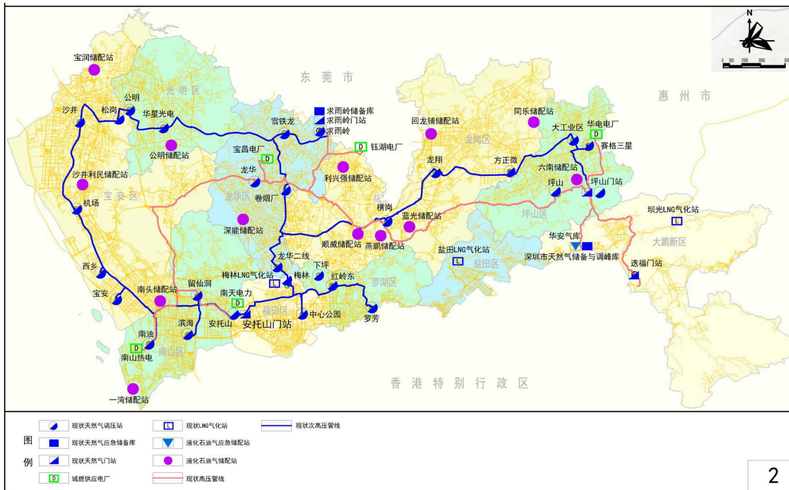
附图 2 城镇燃气场站及高压、次高压管网设施现状布局示意图
