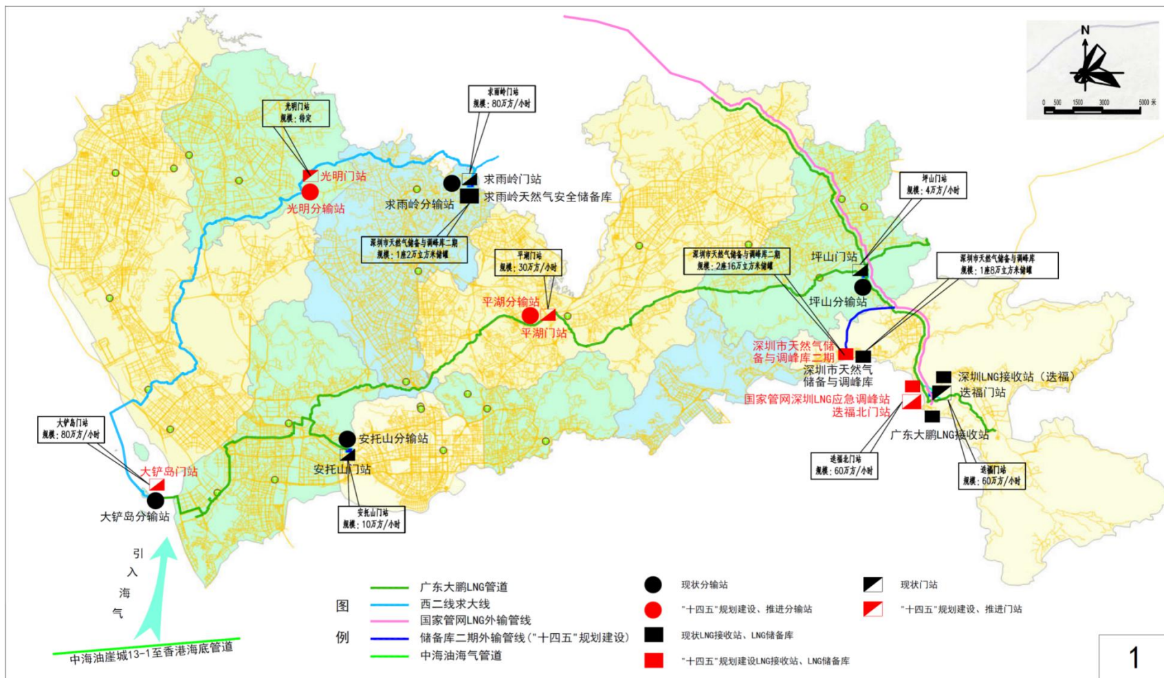
附图 1 深圳市天然气气源布局示意图
