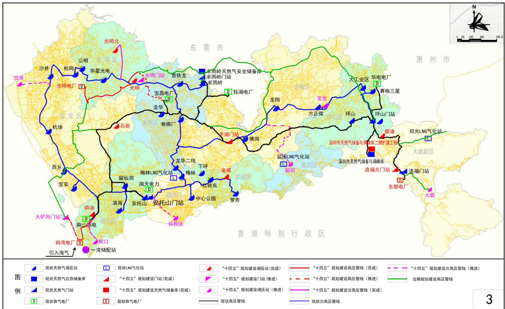
附图3 天然气场站及高压、次高压管网规划布局示意图
